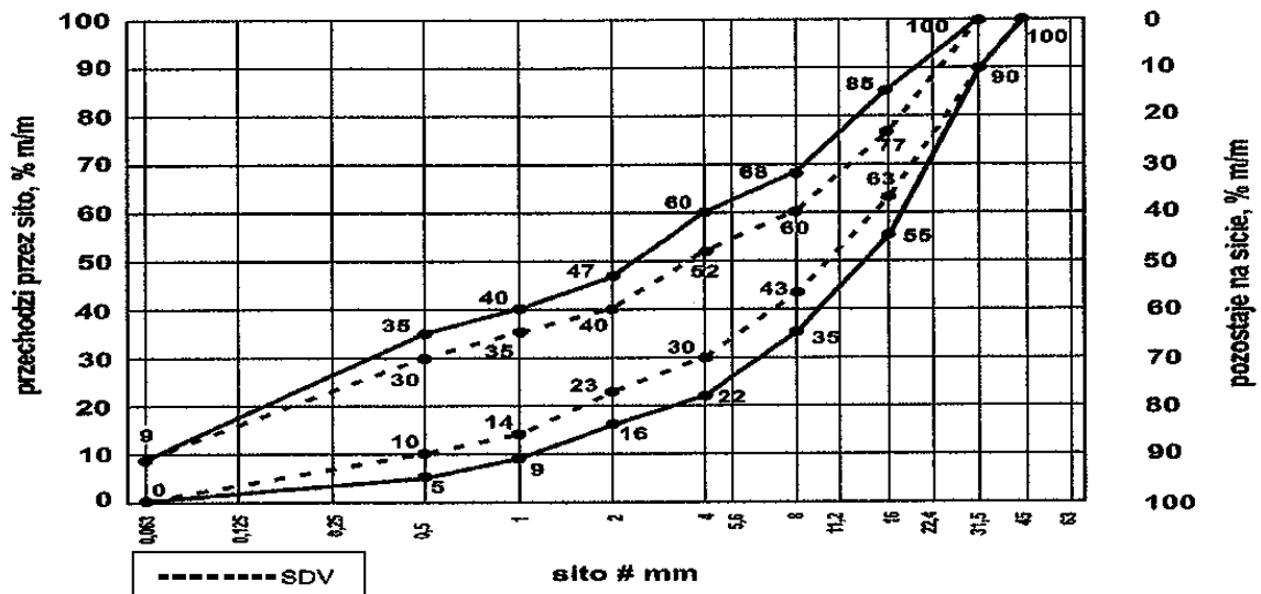
Rys. 1. Krzywe graniczne uziarnienia mieszanki kruszywa 0/31,5 mm do warstw podbudowy zasadniczej
