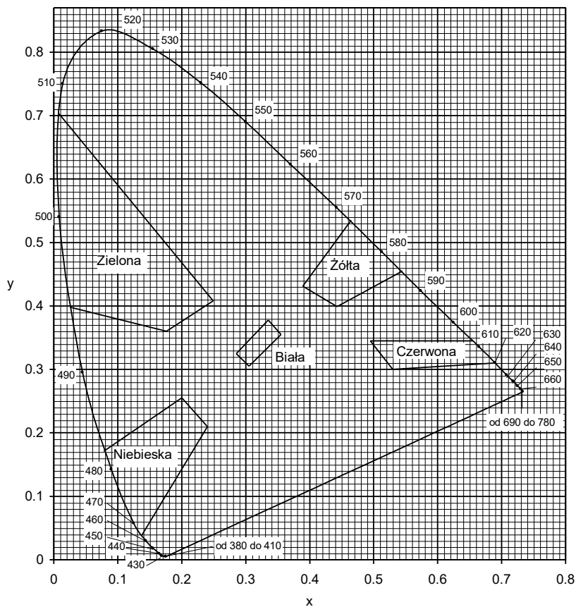
Rys.2. Współrzędne chromatyczości x,y dla barwy żółtej oznakowania
