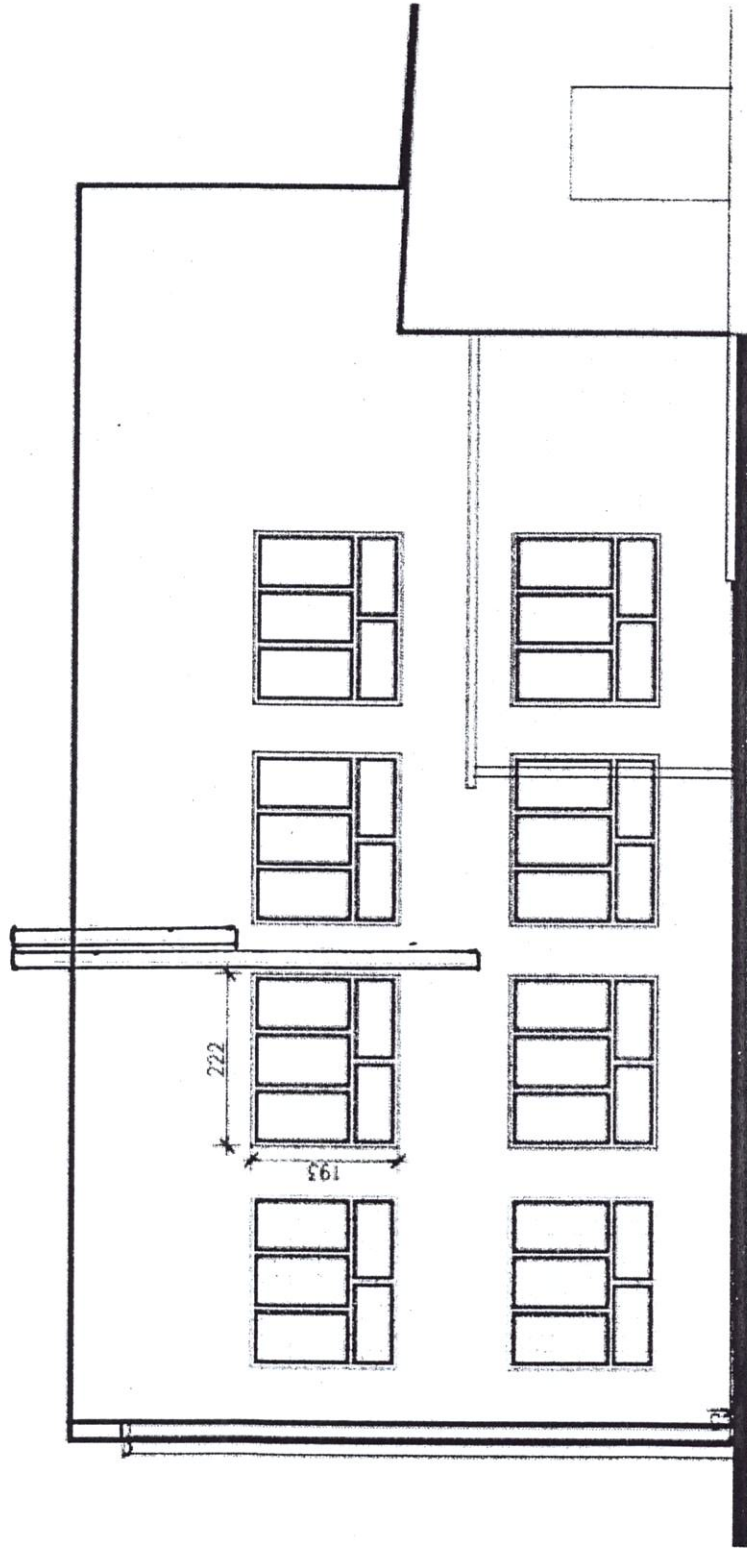
ELEWACJA POŁUDNIOWO WSCHODNIA - SALA 60 60 GI
